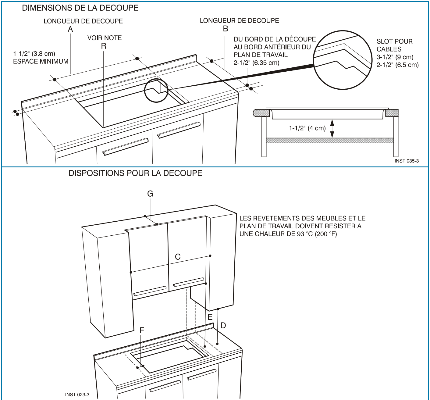
Figure 3. Dimensions pour la découpe
